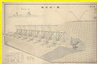
起伏堰ノ圖 第七圖(東西用水酒津陣門)
